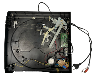
Abb. 02: Antriebskonstruktion
